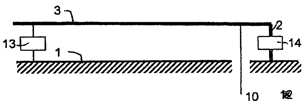
第 5 圖：具有可變反應式元件之倒 F 型天線
